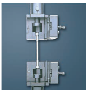
Захват для испытания образцов с сапличками
