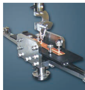
Писпособление для испытания на отрыв
